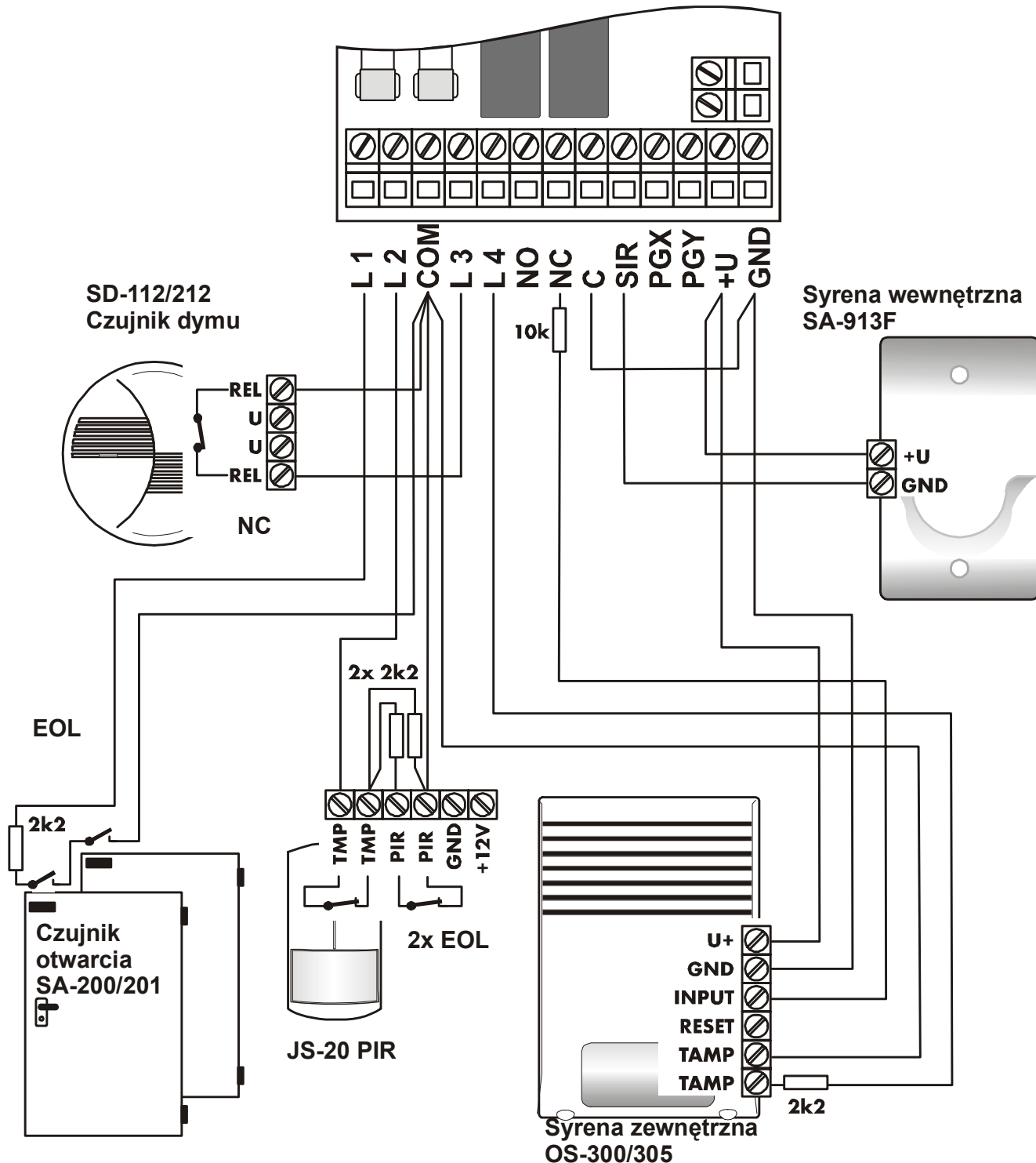
Rys. 1. Połączenia przewodowe
